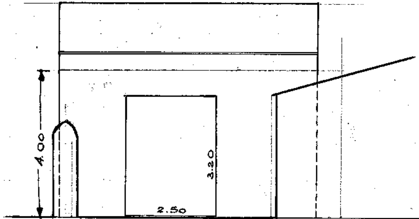
PROSPETTO SCALA 1:100
