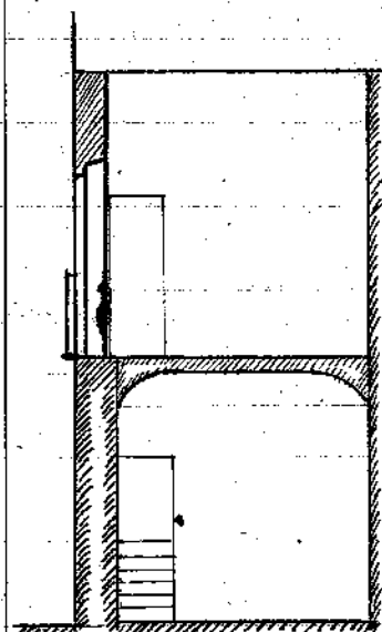
Sezione
